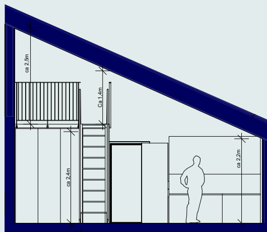
Snitt a-a
