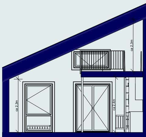
Snitt A-A
