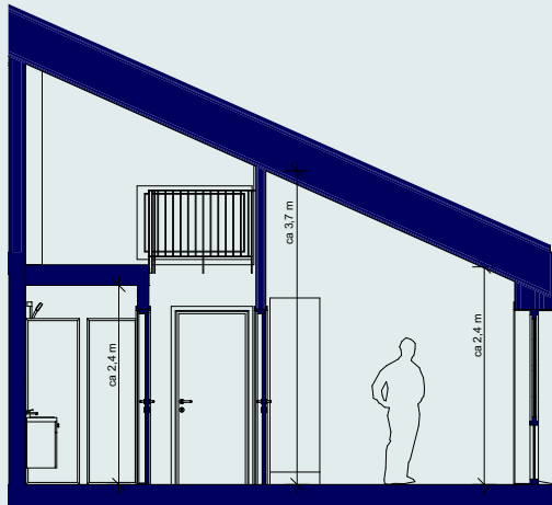
Snitt a-a
