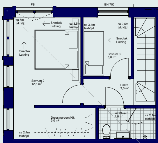
Planlösning övervåning
