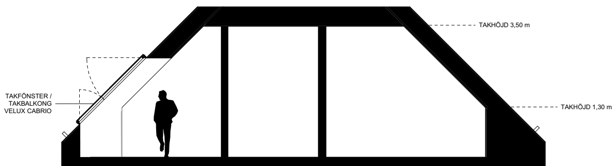
Sektion B 1:100
