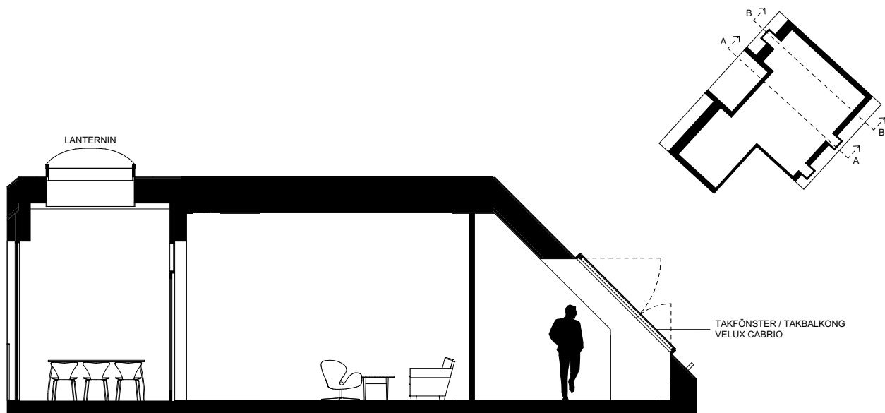
Sektion A 1:100
