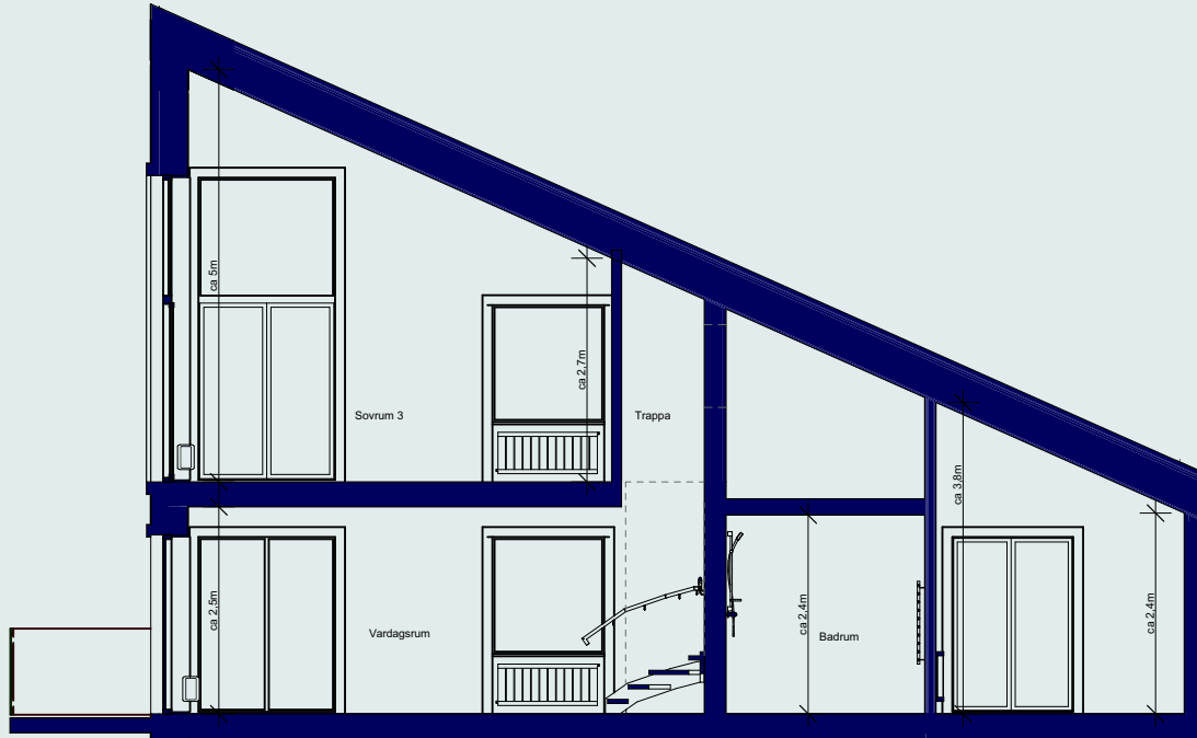
Snitt a-a
