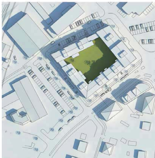
Fig 31, Sommarsolstånd kl 9.00
