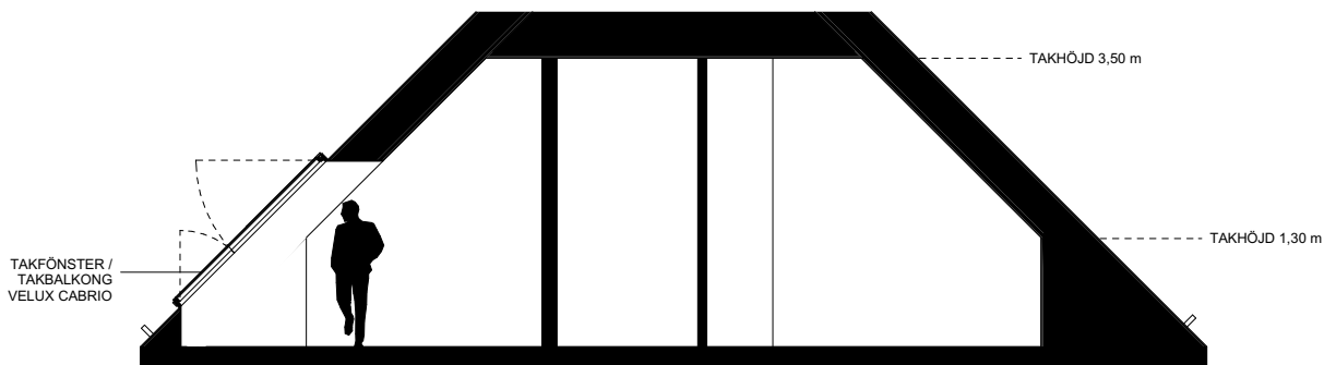
Sektion B 1:100
