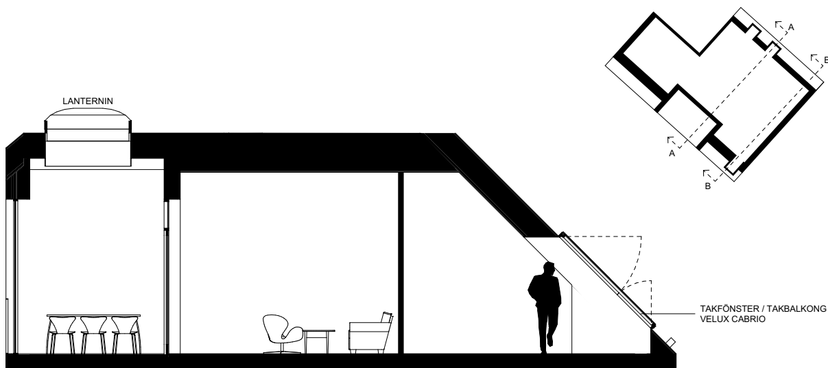
Sektion A 1:100
