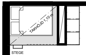
Loftplan
