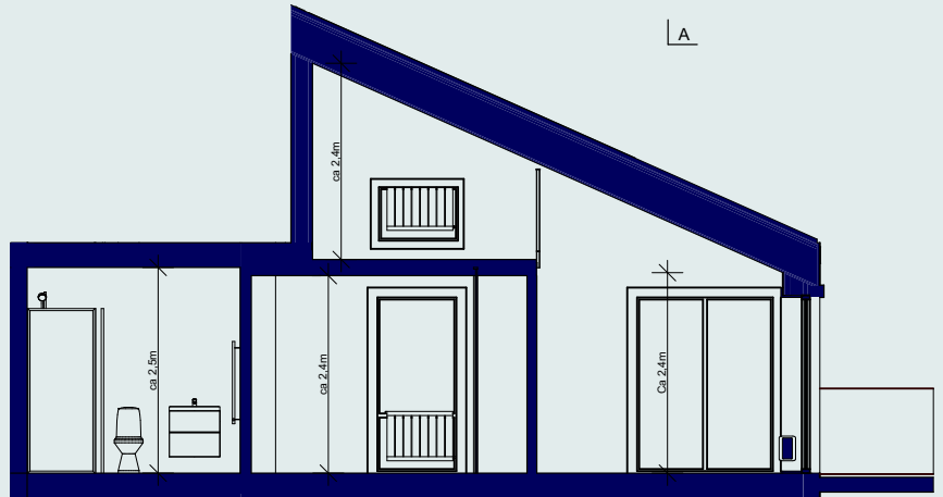
Snitt A-A
