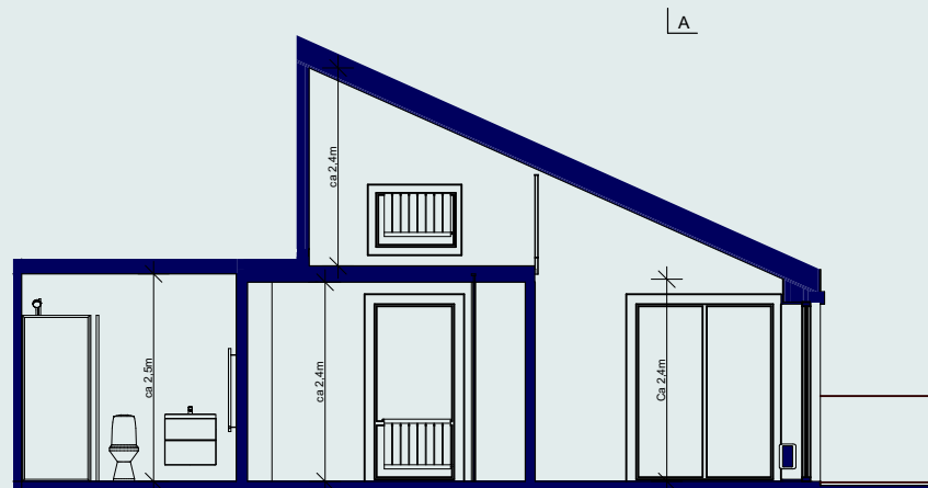
Snitt A-A
