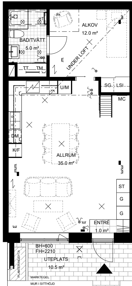
VÅNING 0
