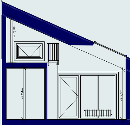
Snitt A-A
